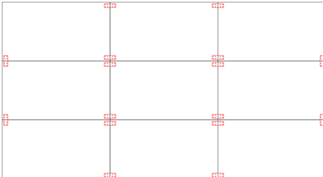
Схема установки соединительных пластин. Вид с тыльной стороны видеостены
