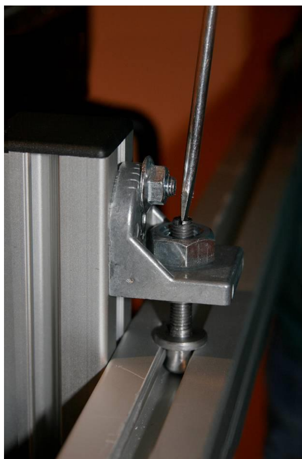
Регулирование вертикального расположения панели
